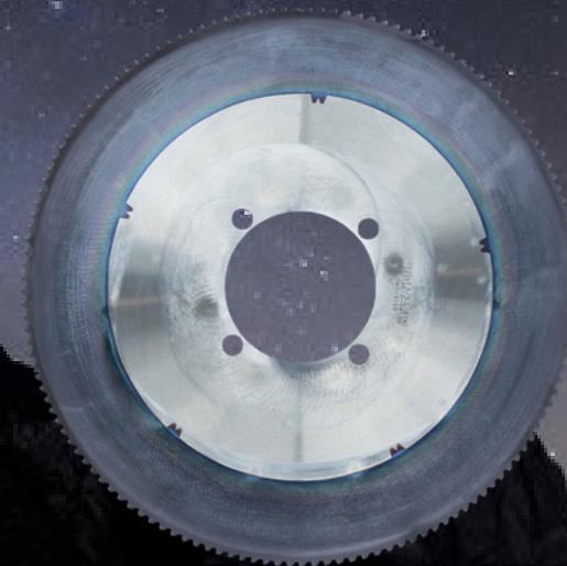
Lama dopo il processo InfinityCut
