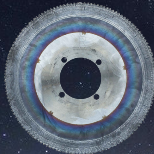
Lama prima del processo InfinityCut
